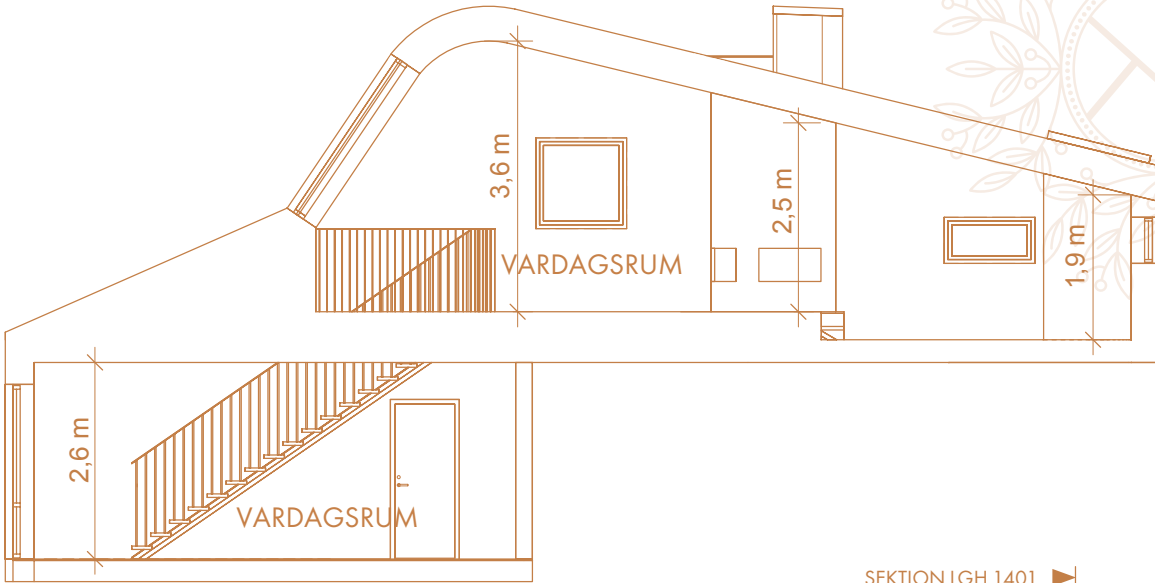
SEKTION LÄGENHET 1401
